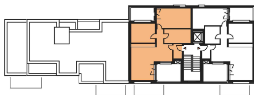
Staffelgeschoss
