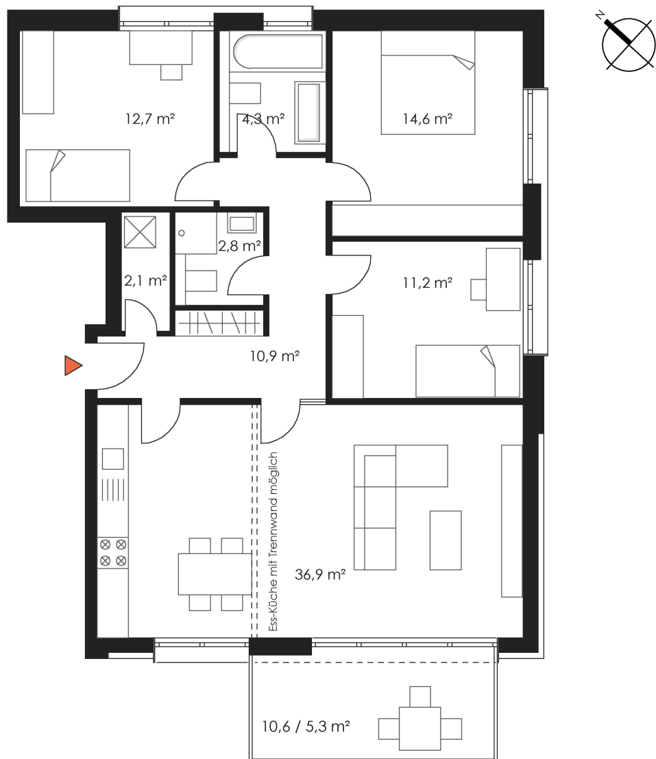
Grundrissvorschlag
