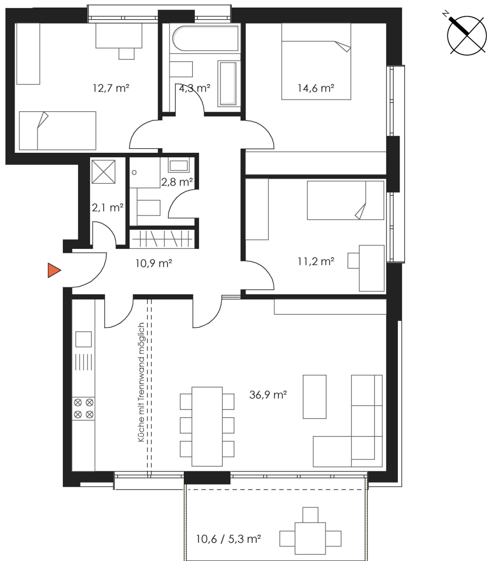
Grundrissvorschlag
